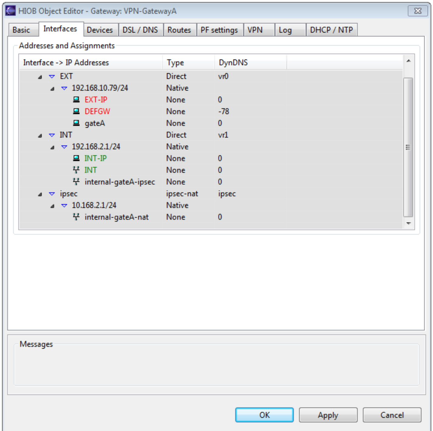
Bild 8.3 VPN-GatewayA
