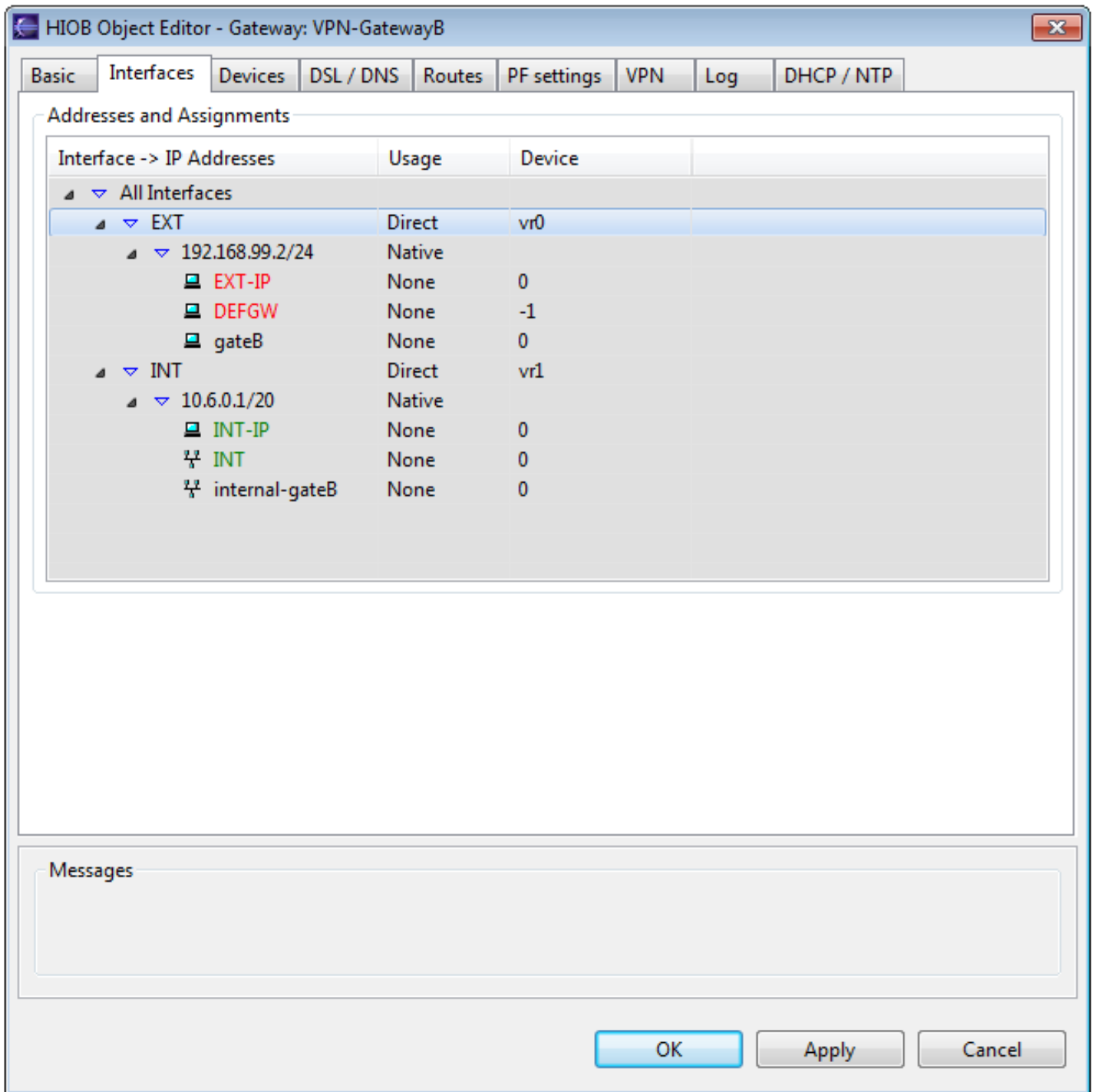
Bild 8.4 VPN-GatewayB
