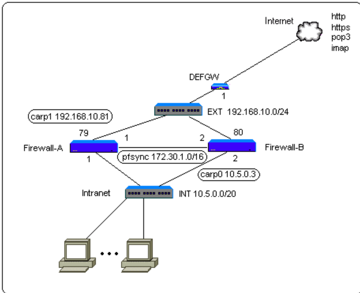
Bild 7.1 Firewall-Cluster
